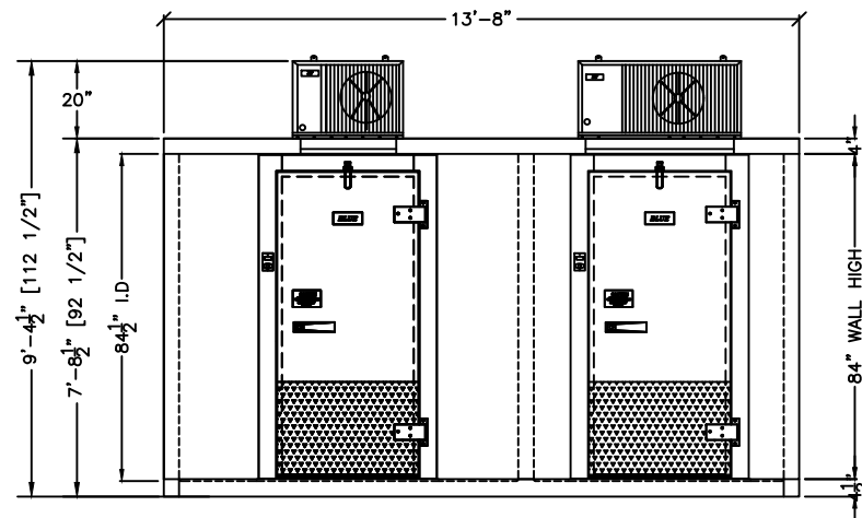
1 ELEVATION SCALE: 1/4"=1'-0"
