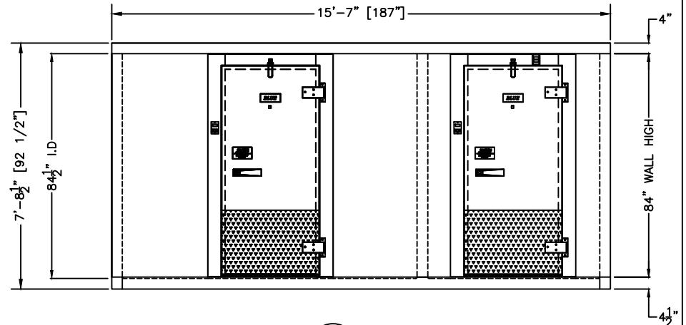
1 ELEVATION SCALE: 1/4"=1'-0"
