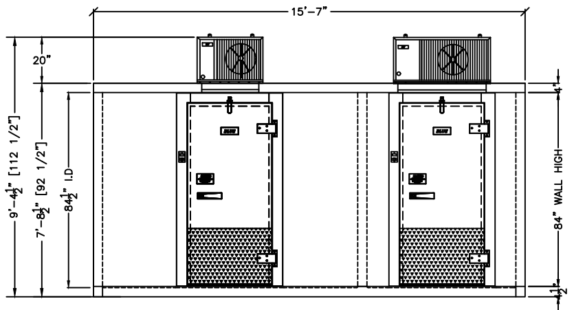
1 ELEVATION SCALE: 1/4"=1'-0"
