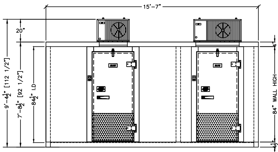
1 ELEVATION SCALE: 1/4"=1'-0"
