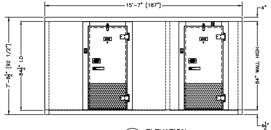
1 ELEVATION SCALE: 1/4"=1'-0"
