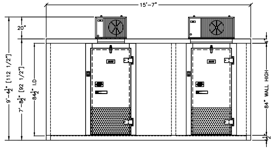
1 ELEVATION SCALE: 1/4"=1'-0"
