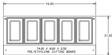
Plan View EHEI74C
