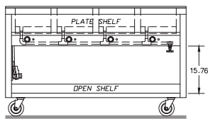
Elevation View EHEI60C
