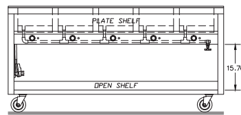
Elevation View EHEI74C
