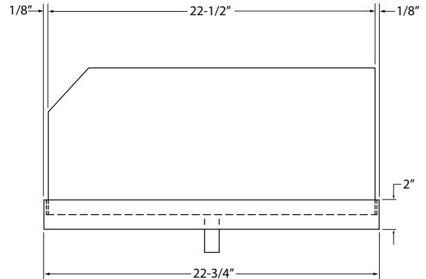
24" Deep GDU
