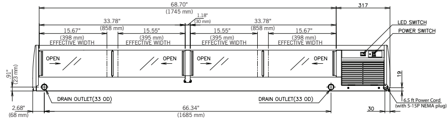
HNC-210-BA-L-SLH
