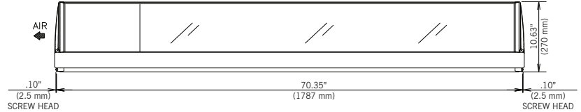
HNC-180-BA-L-SLH
