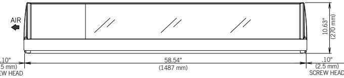
HNC-150-BA-L-SLH
