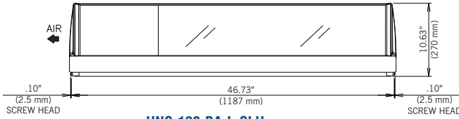
HNC-120-BA-L-SLH
