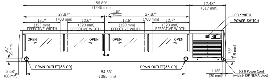
HNC-180-BA-L-SLH
