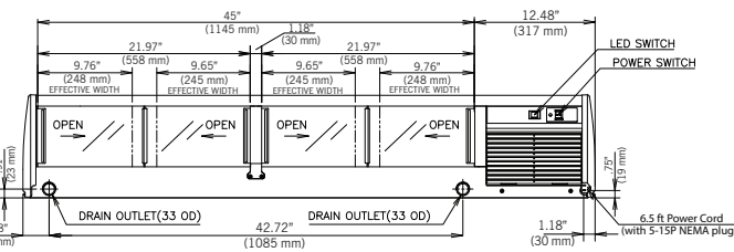
HNC-150-BA-L-SLH
