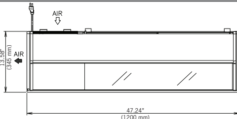
HNC-120-BA-L-SLH
