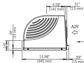
HNC-150-BA-L-SLH
