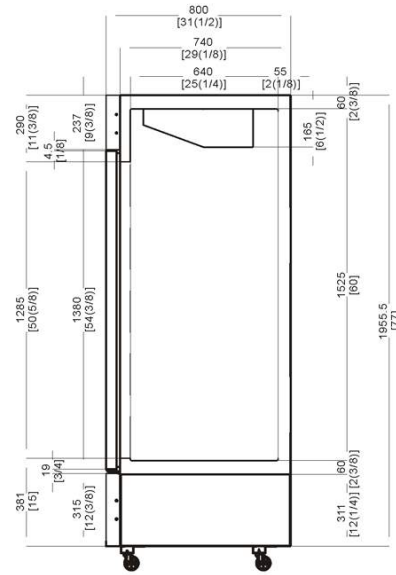
SIDE VIEW ( 1,2,3 DOOR MODELS)
