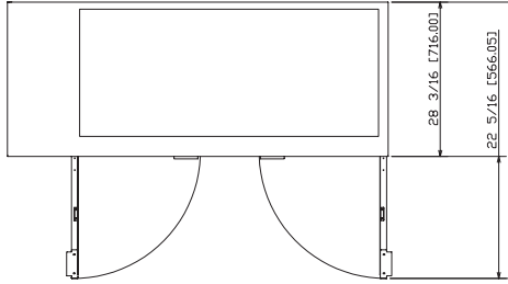
TOP NLBB69
