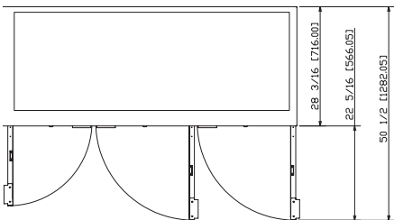
TOP NLBB79
