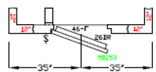
OPTION A DOOR SWING
