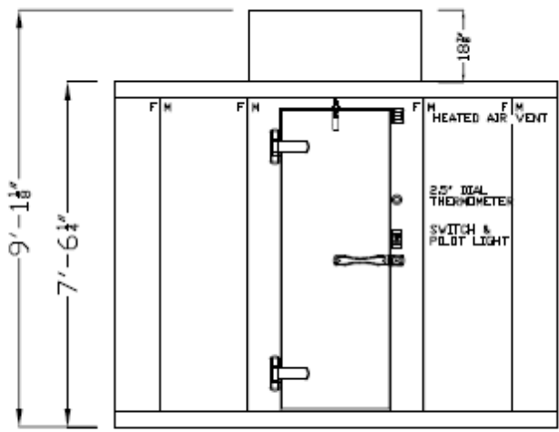
DOOR ELEVATION 46x7DS 26x78 DR P-P-FRZ STD THRESHOLD DETAIL 02
